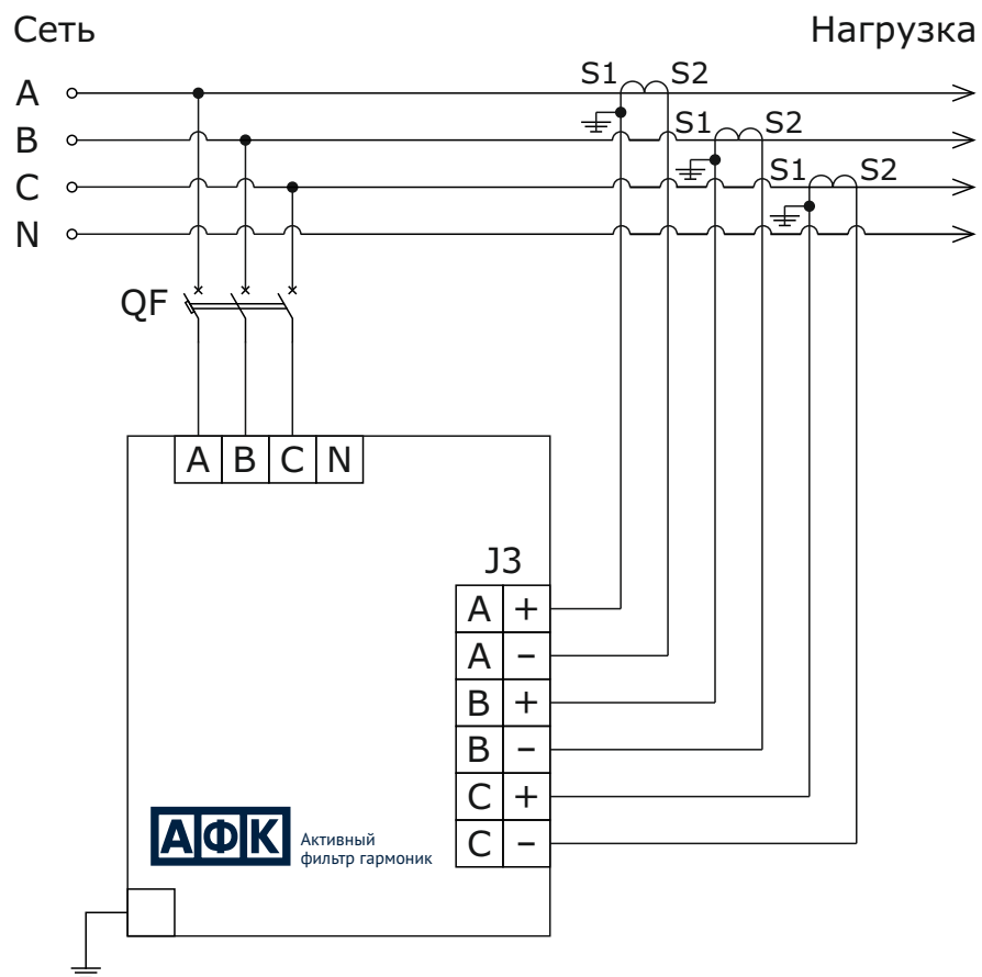
Рисунок 3 - Схема подключения ТТ со стороны нагрузки (без нейтрали)
