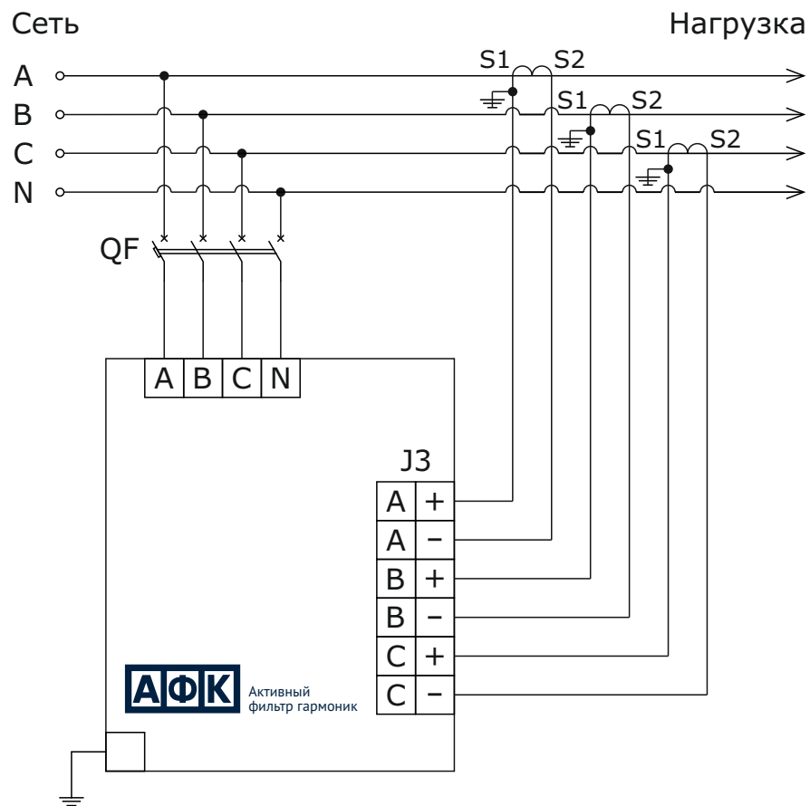
Рисунок 2 - Схема подключения ТТ со стороны нагрузки (с нейтралью)
