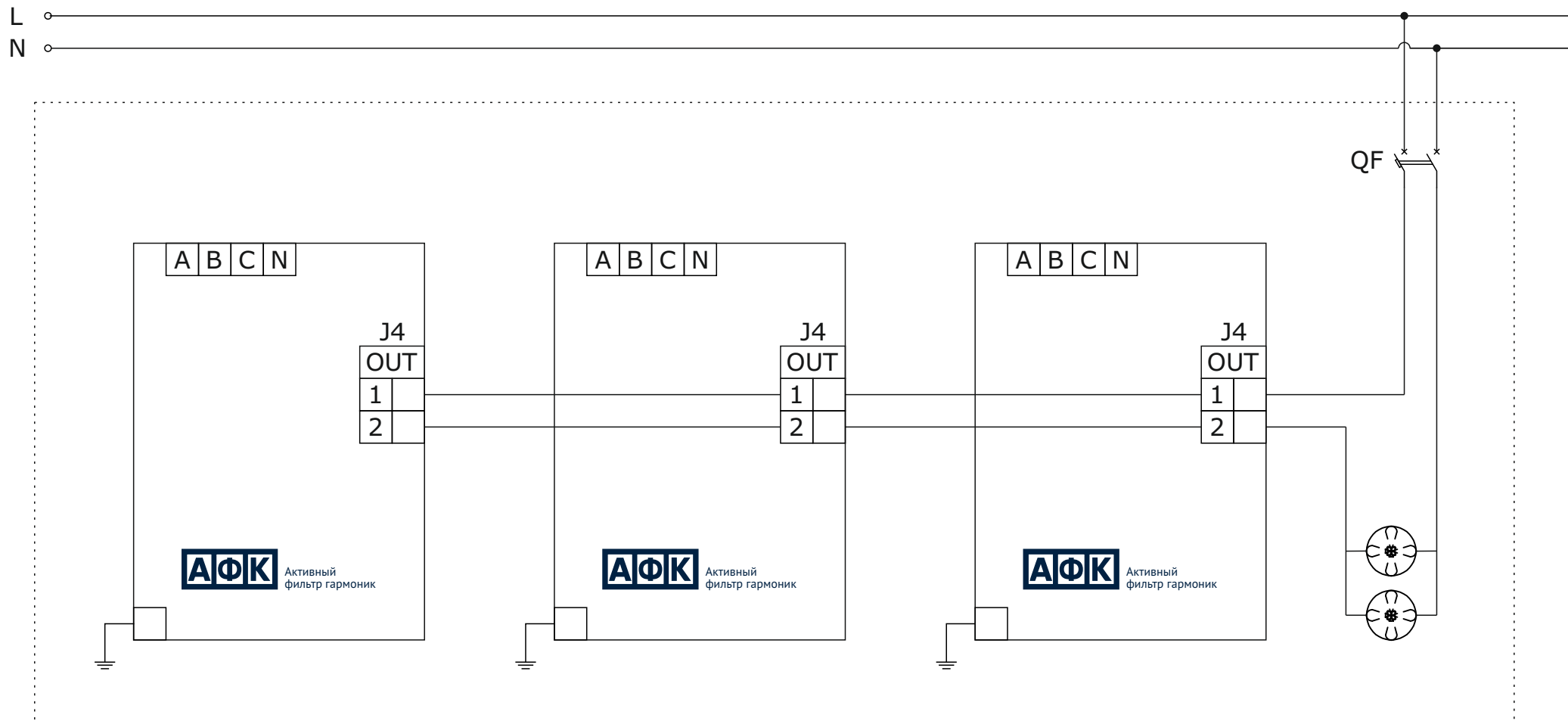
Рисунок 7 - Подключение шкафного вентилятора охлаждения при параллельном режиме работы
