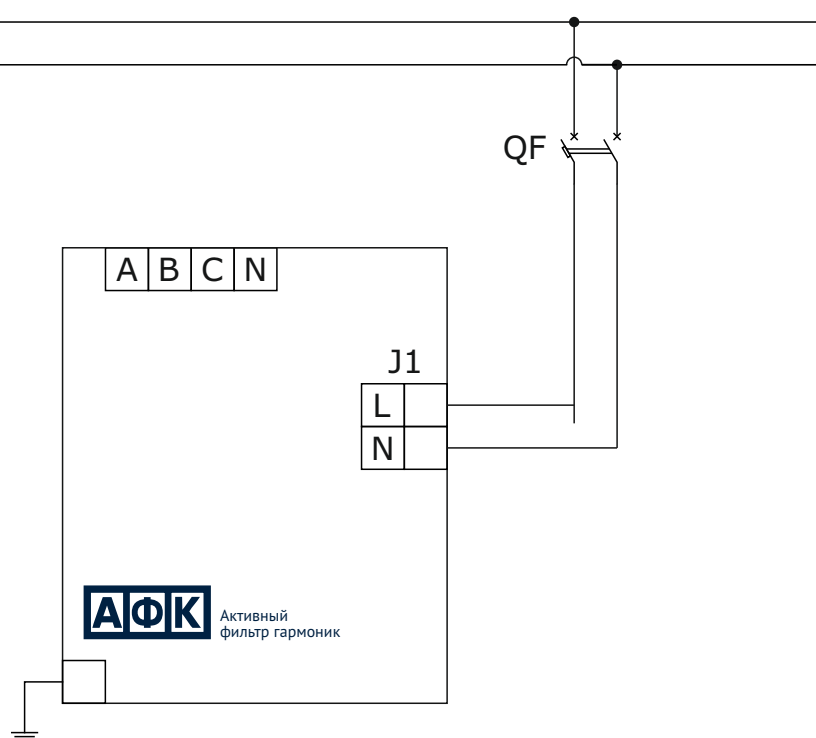
Рисунок 1 - Схема подключения питания цепей управления
